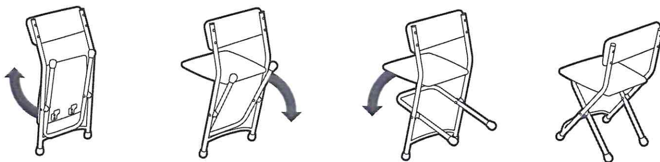
(рис. 4) Схема раскладывания стула с мягкой обивкой
